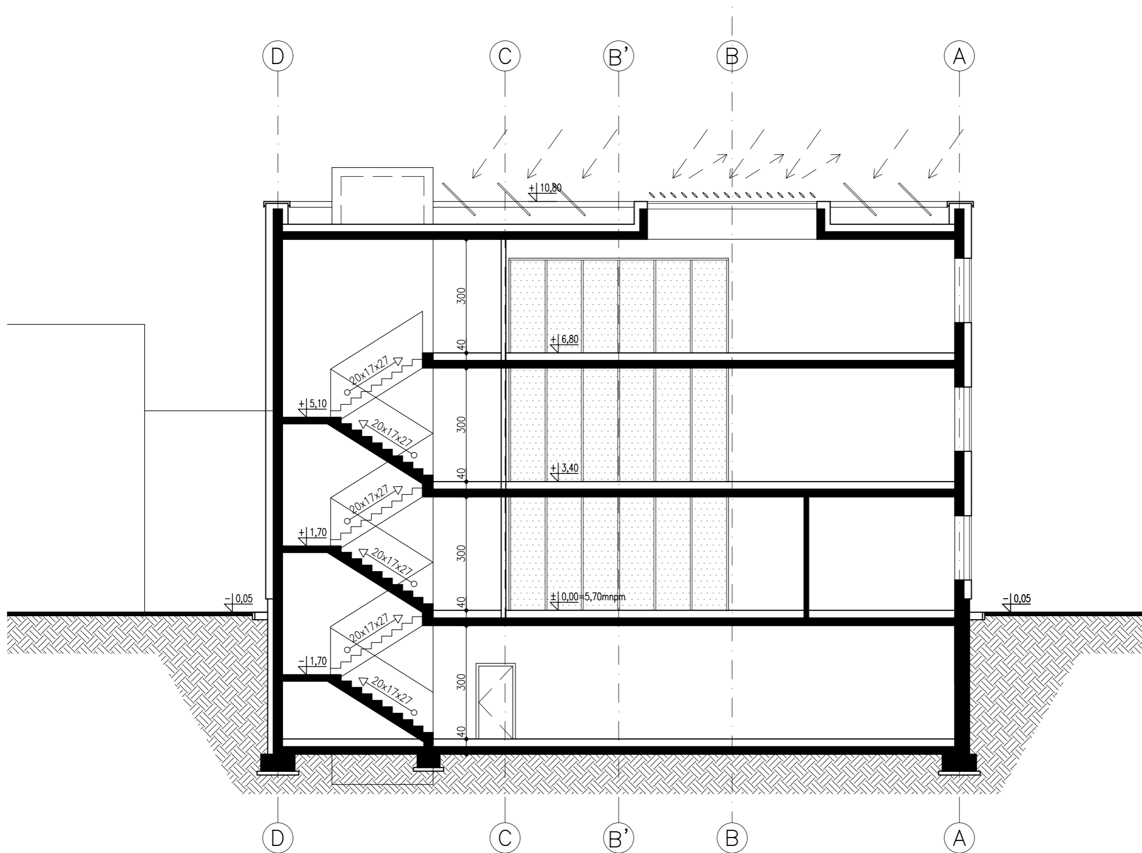
PRZEKRÓJ 1-1, SKALA 1:100
