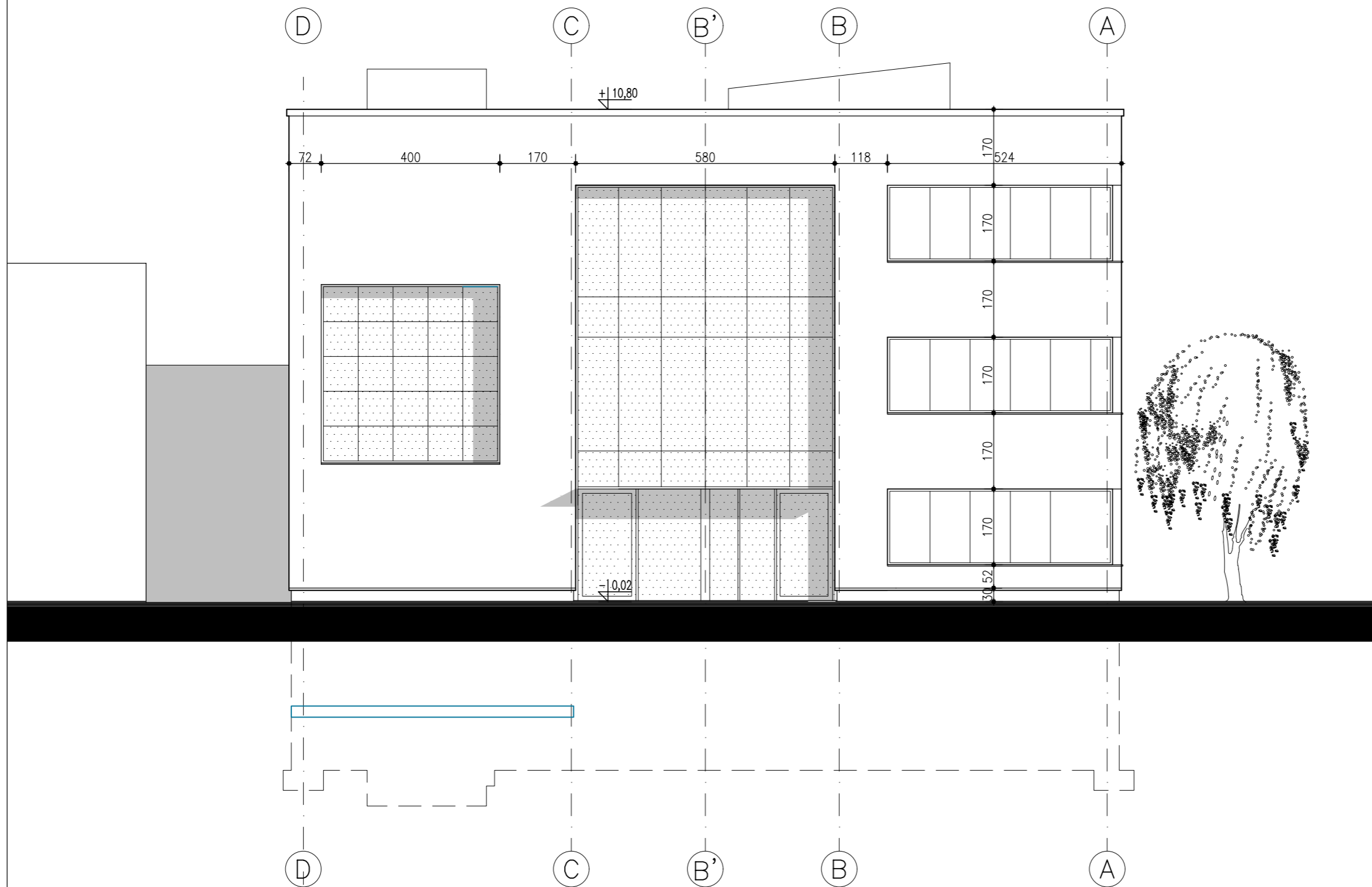
ELEWACJA ZACHODNIA (FRONTOWA), SKALA 1:100
