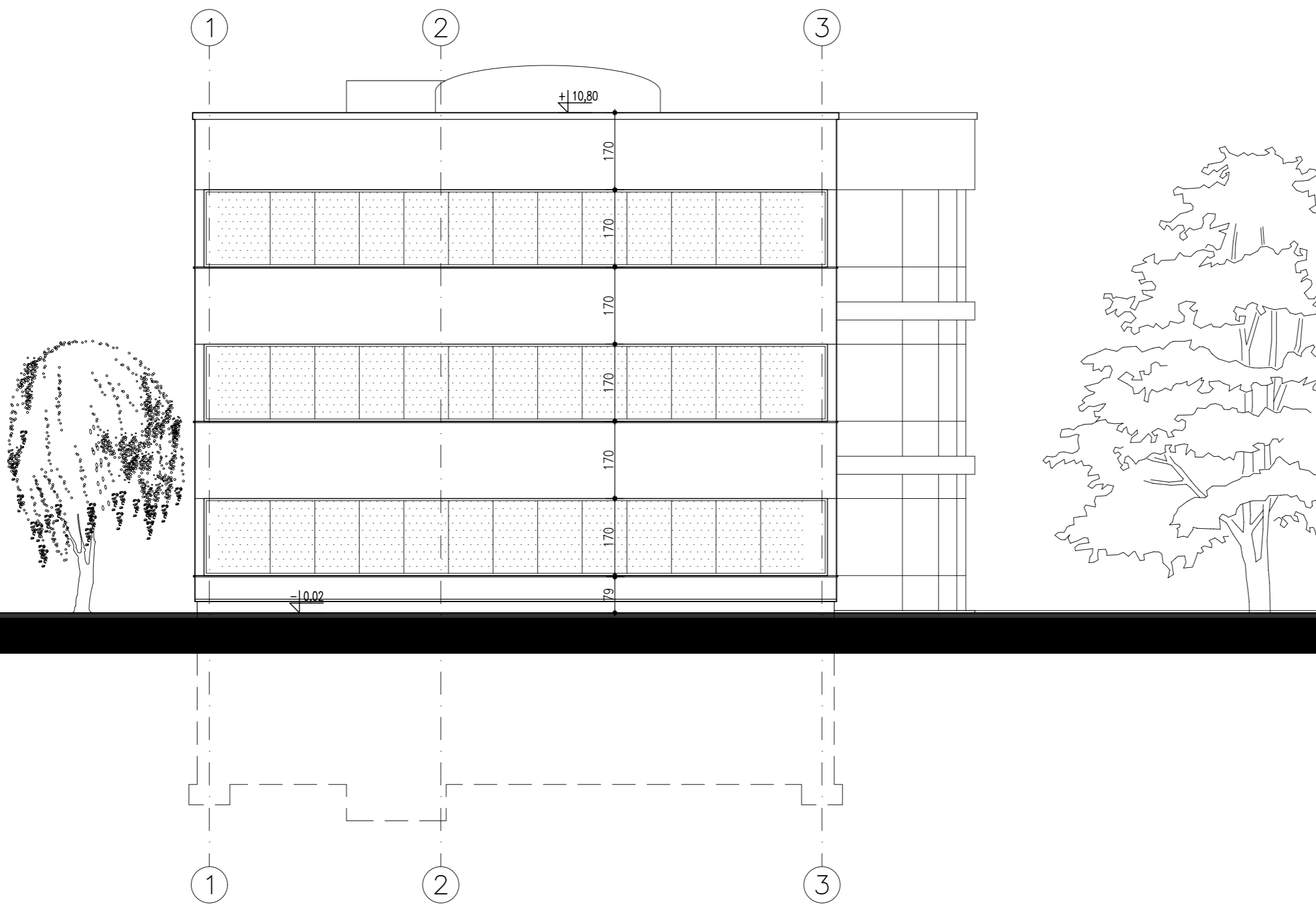
ELEWACJA POŁUDNIOWA, SKALA 1:100
