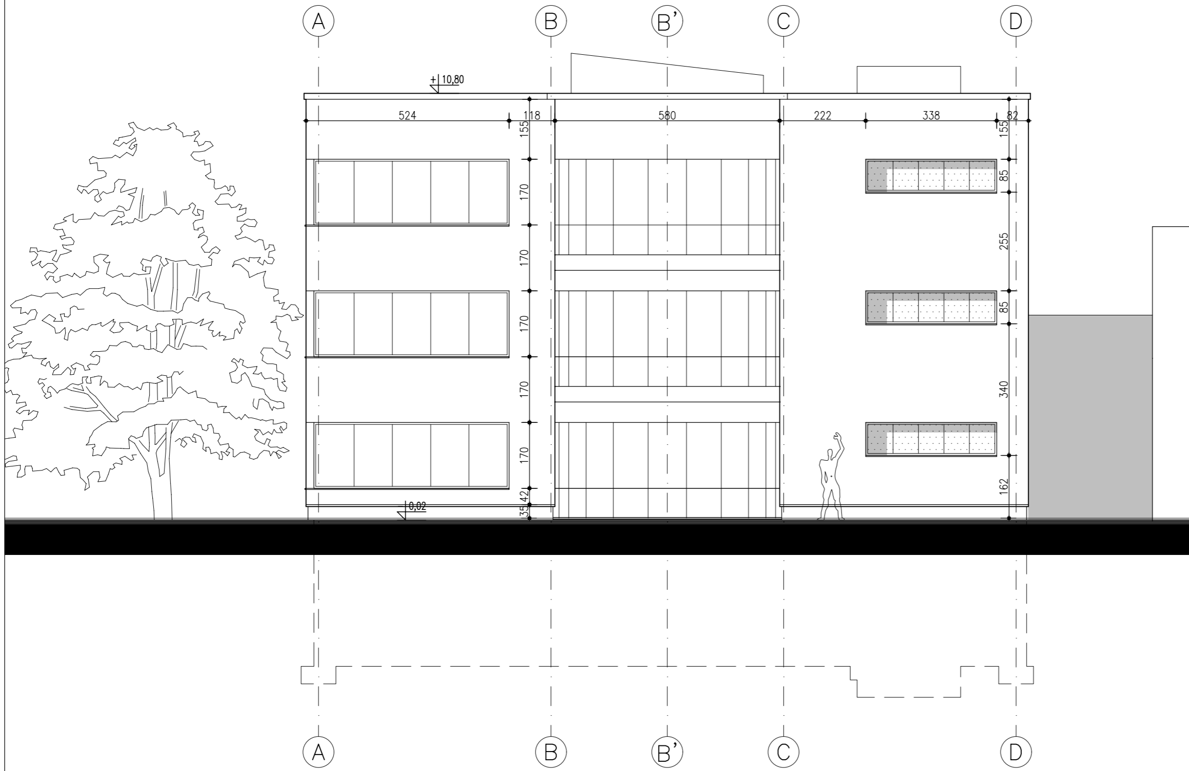
ELEWACJA WSCHODNIA, SKALA 1:100
