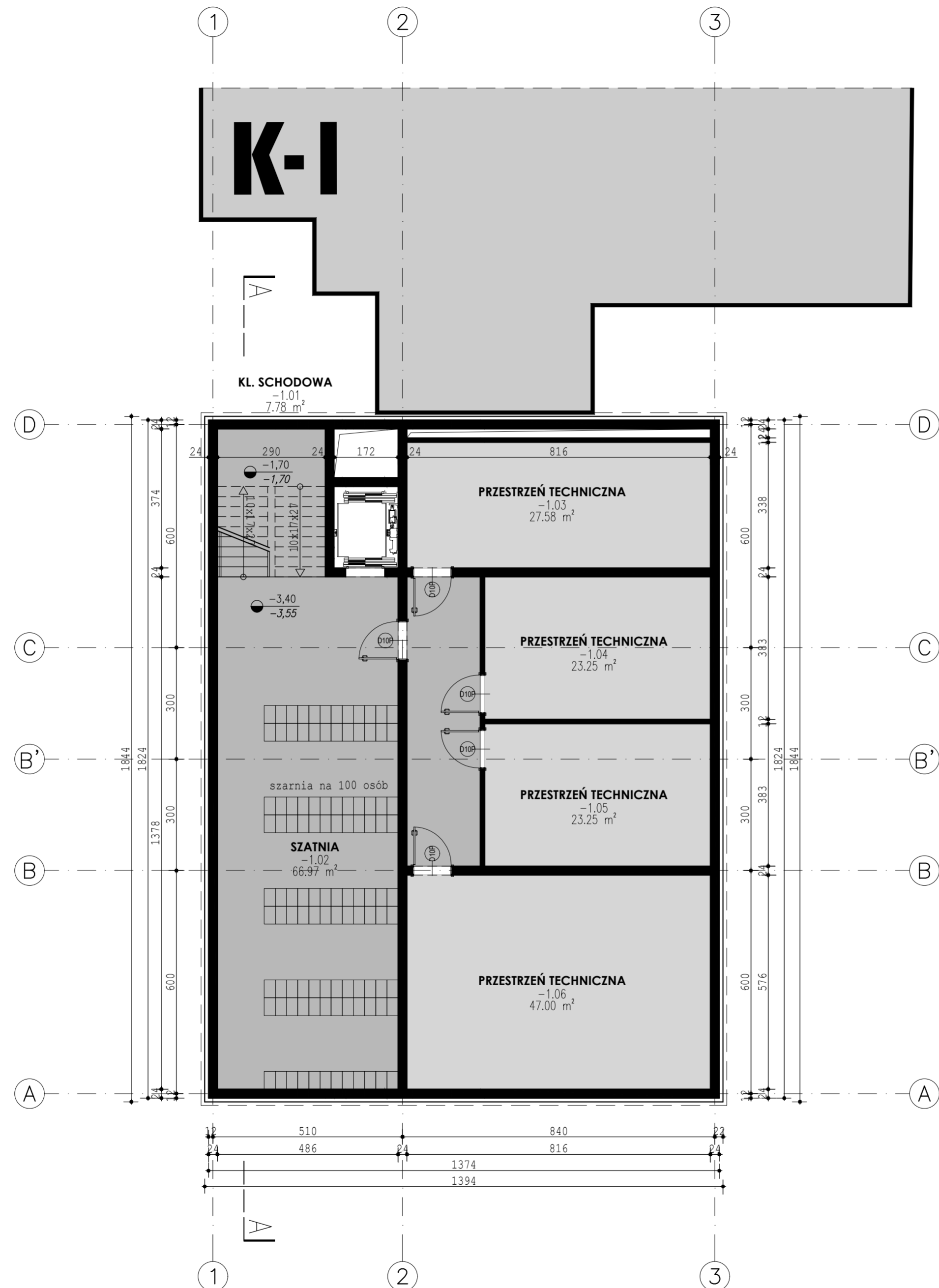
RZUT KONDYGNACJI K-1, SKALA 1:100
