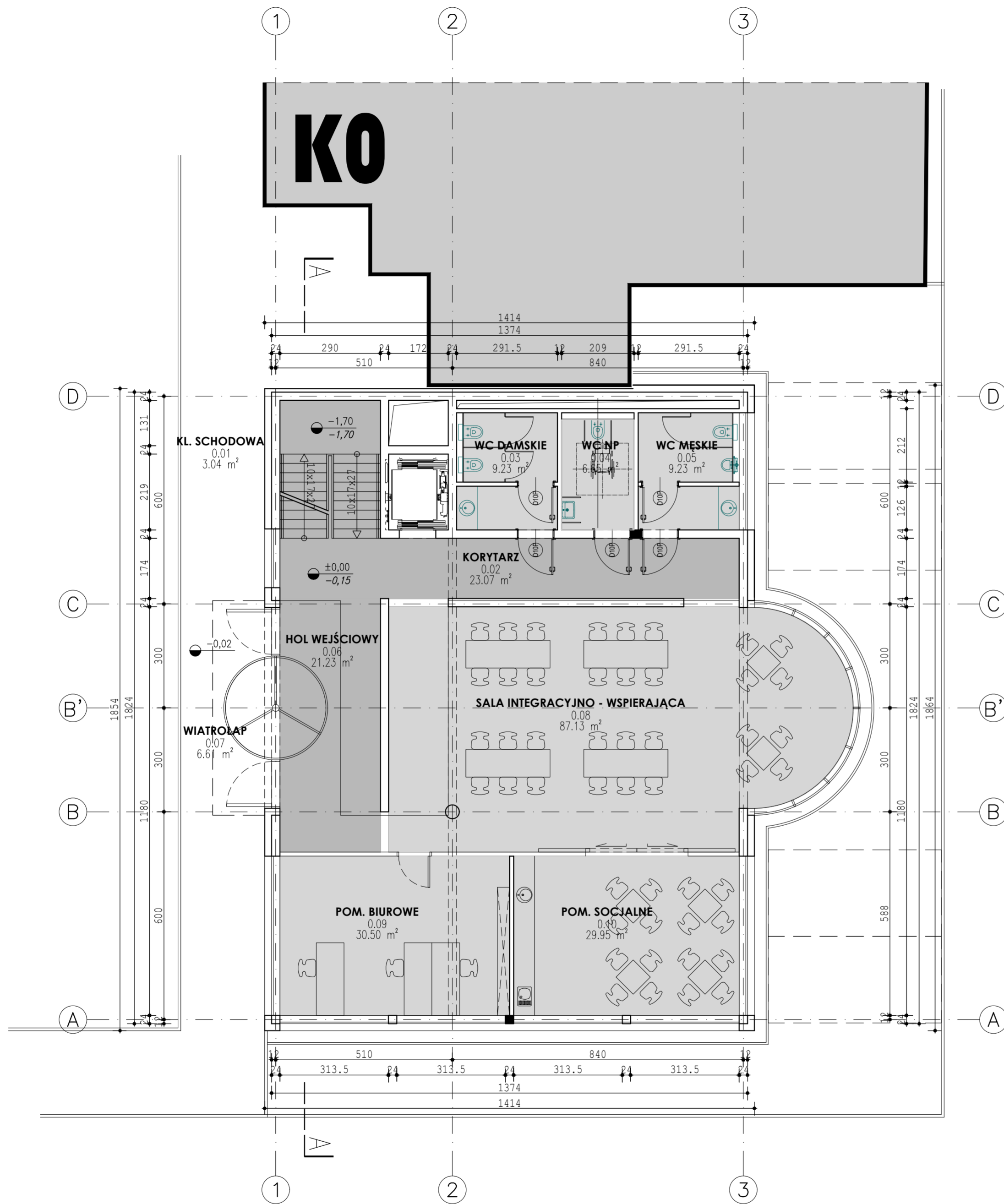
RZUT KONDYGNACJI K0, SKALA 1:100 CZEŚĆ INTEGRACYJNO - WSPIERAJĄCA CZEŚĆ DORADCZO - PROMOCYJNA
